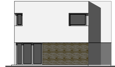
elewacja południowa
